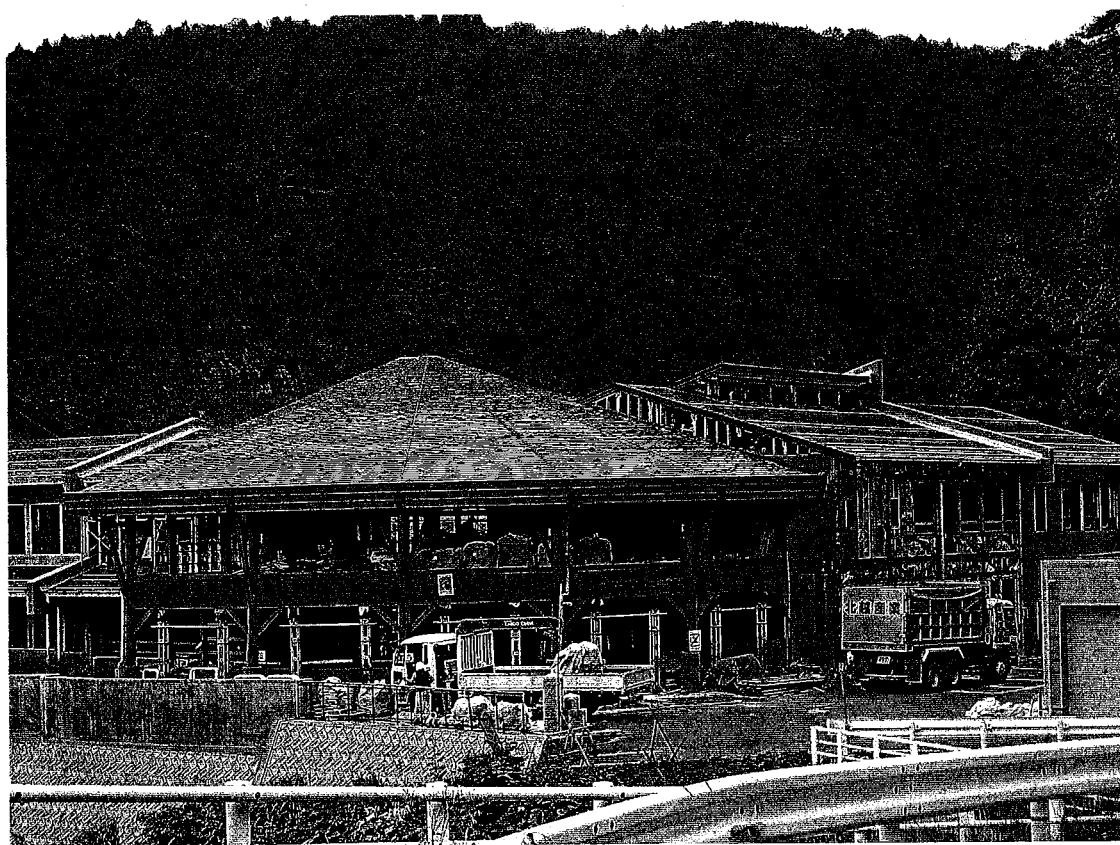
解体工事に向けての準備 平成17年7月6日(水) 撮影
